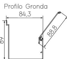
Profilo Compensatore posteriore lamelle
