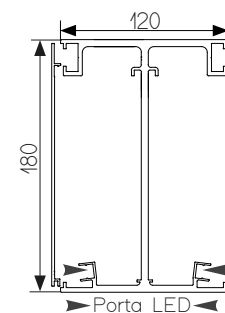
Guida portante con carter di chiusura
